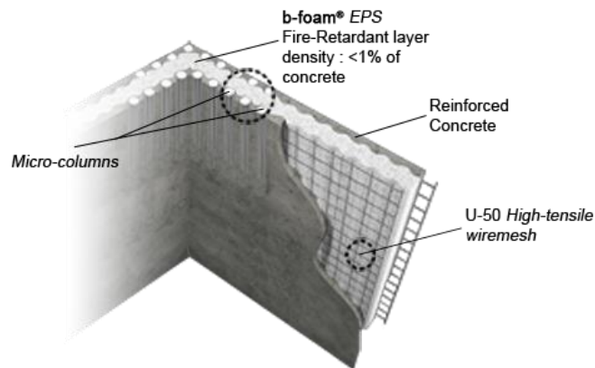
Gambar 4. Lapisan EPS Sumber : Dokumentasi Pribadi
